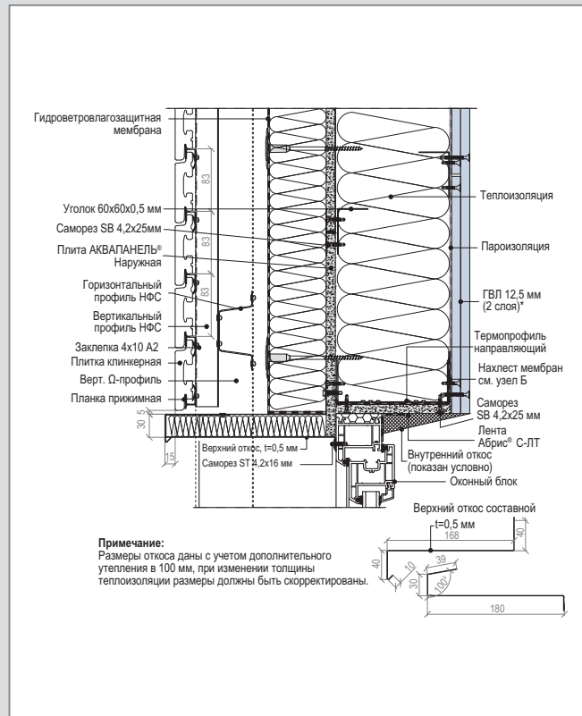
A 5 – WM 111 (4а 100) С. Верхнее примыкание к оконному блоку
