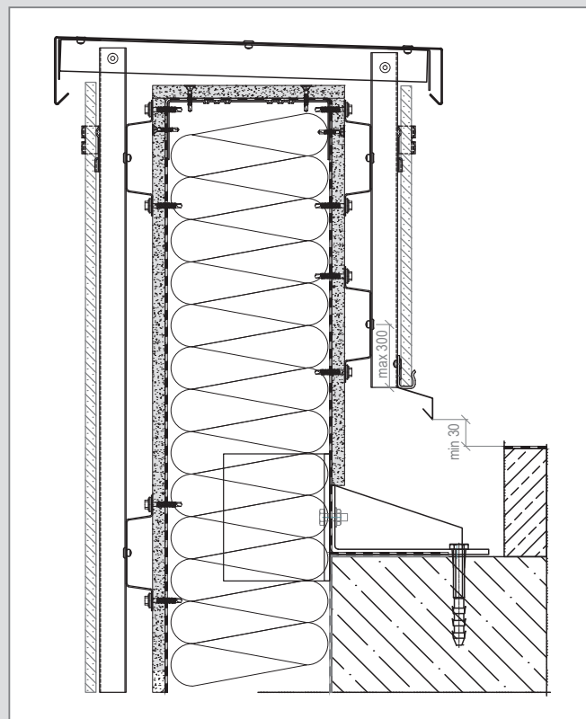
D 4 – WM 112 (2) С. Крепление к плите покрытия. Паралет
