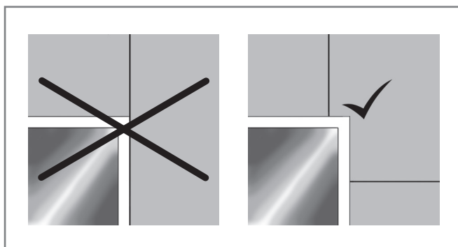
Рис. 23. Крепление плит в области проема
