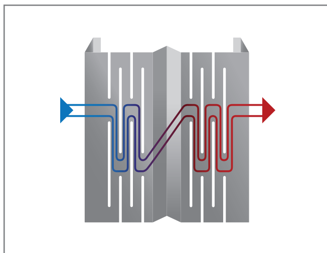
Рис. 13. Перфорация термопрофиля. Принцип движения теплового потока
