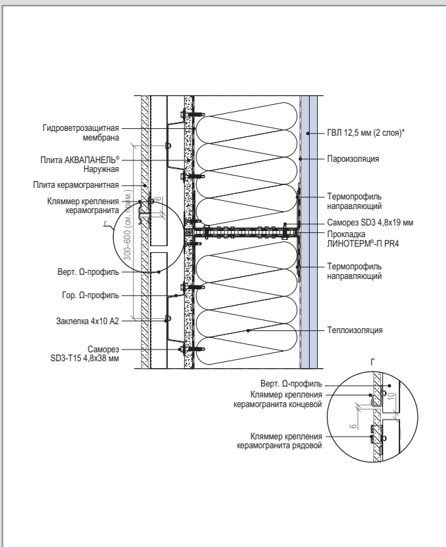
C 6 – WM 112 (2) С. Горизонтальный стык смежных модулей
