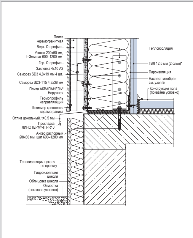
C 5 – WM 112 (2) С. Примыкание к фундаменту. Вариант 2
