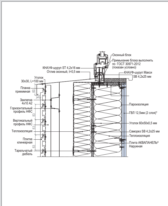
A 4 – WM 111 (4а 100) С. Нижнее примыкание к оконному блоку
