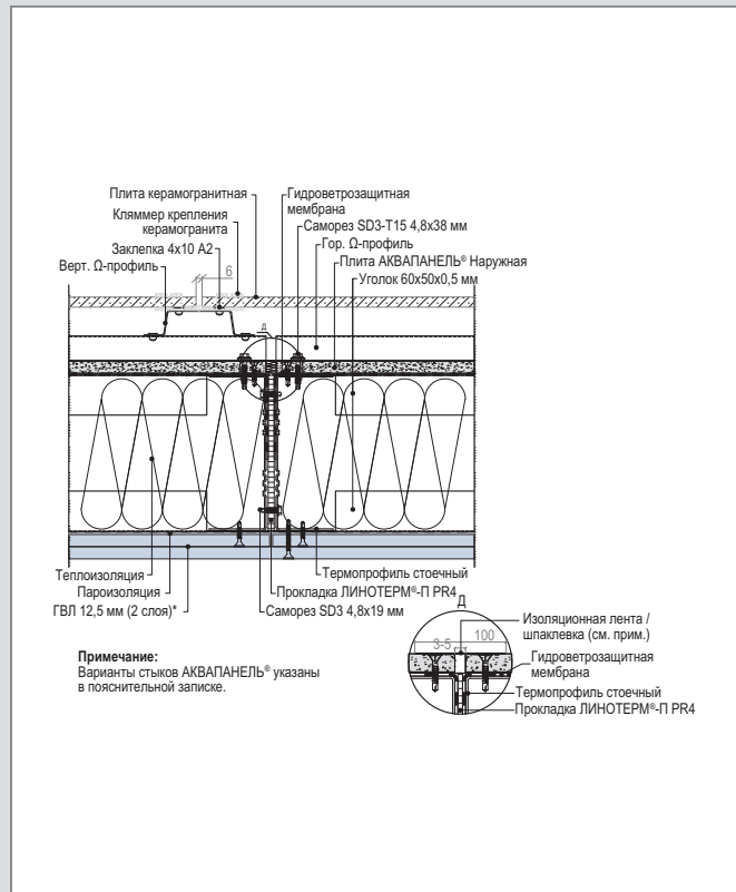
C 6 – WM 112 (2) С. Вертикальный стык смежных модулей
