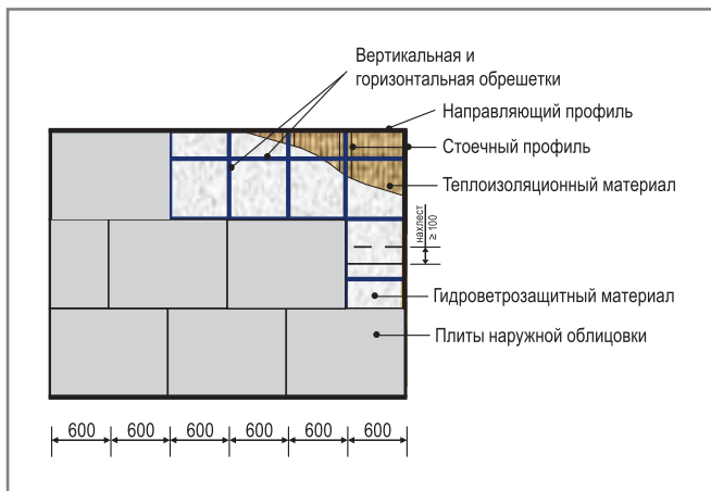
Рис. 22. Крепление наружной обшивки к каркасу
