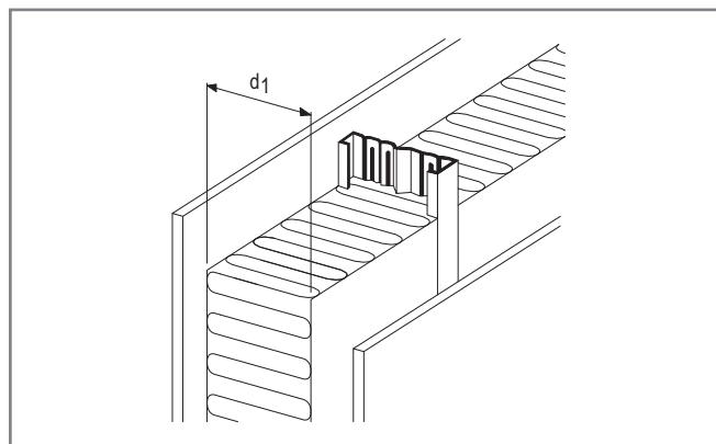
Рис. 14. Толщина утепляющего слоя наружной КОС с применением ЛСТК
