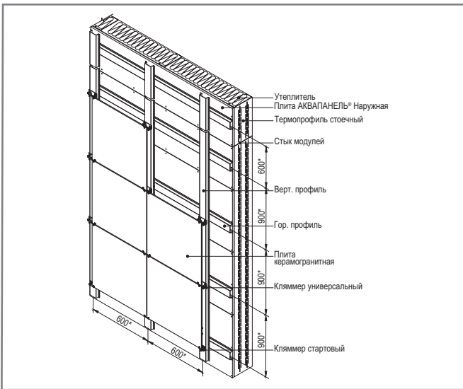
Рис. 1. Общий вид наружной каркасно-обшивной стены (КОС) с каркасом из ЛСТК
