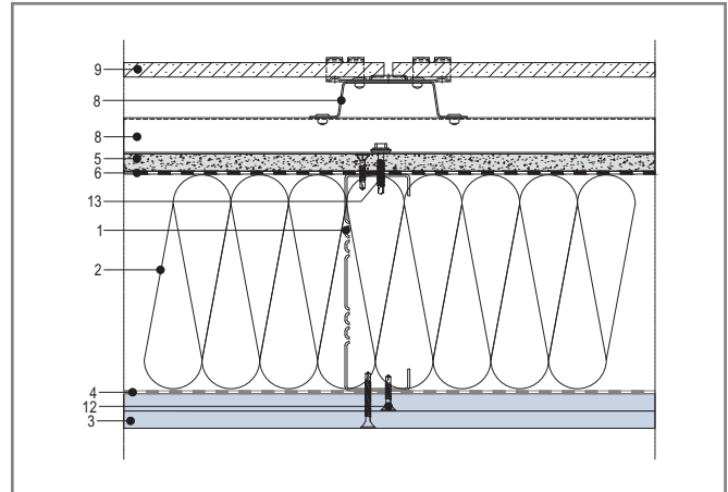
Рис. 7. Тип № 2. Схема конструктивного исполнения наружной несущей КОС с зазором с внешней стороны (расшифровку цифровых обозначений см. в табл. 1)
